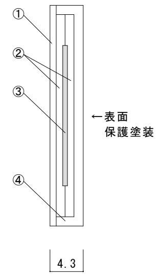
断面図 【 a-a' 】
