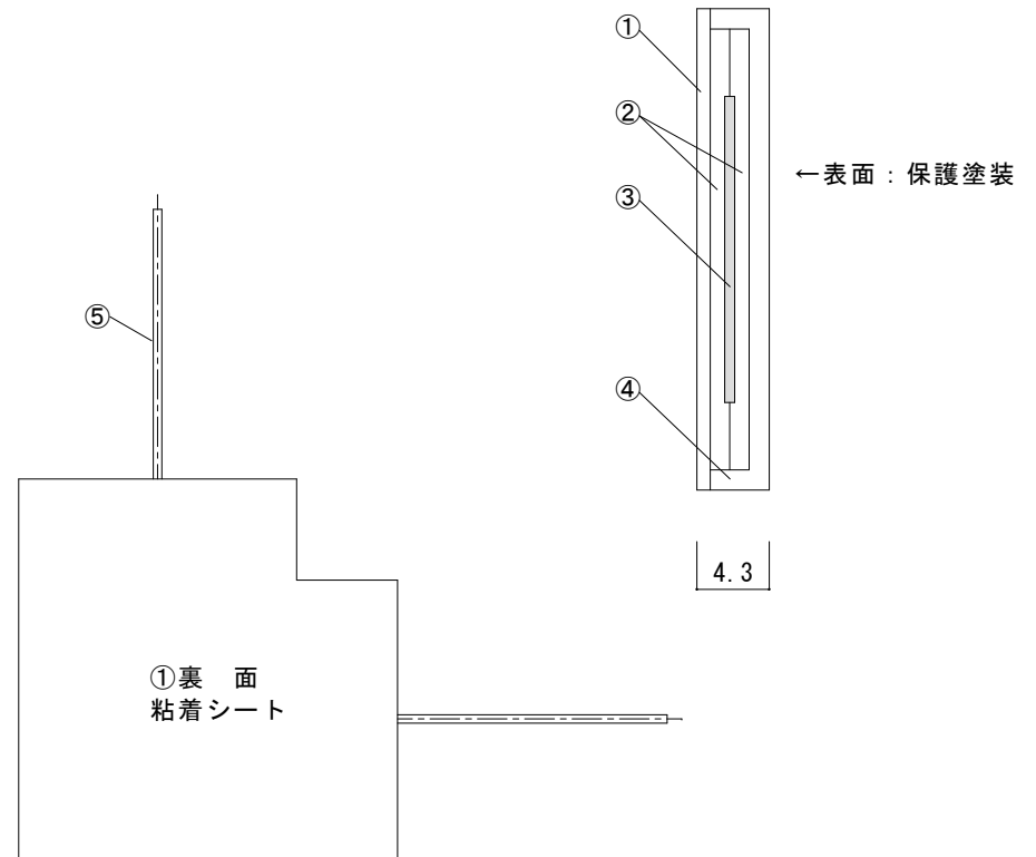
断面図 【 a-a' 】
