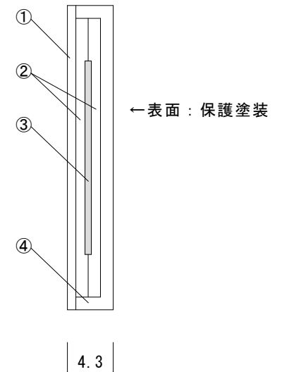
断面図 【 a-a' 】
