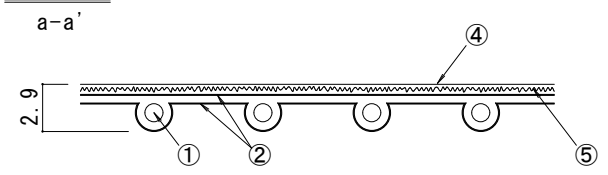
断面図
