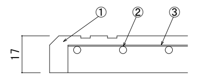
拡大断面図
